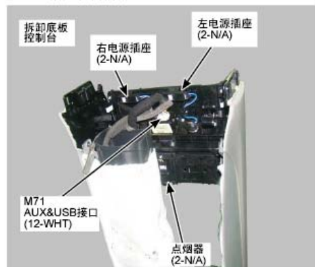
144. 底板控制台前部
